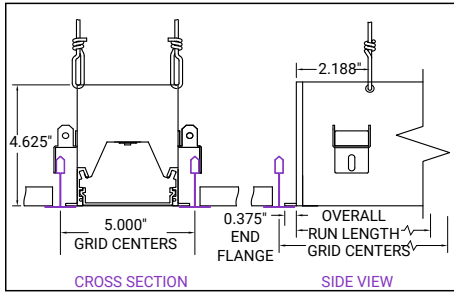
9/16 Tee (FTG)
