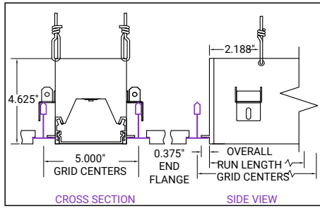
9/16 Tegular (FTT)
